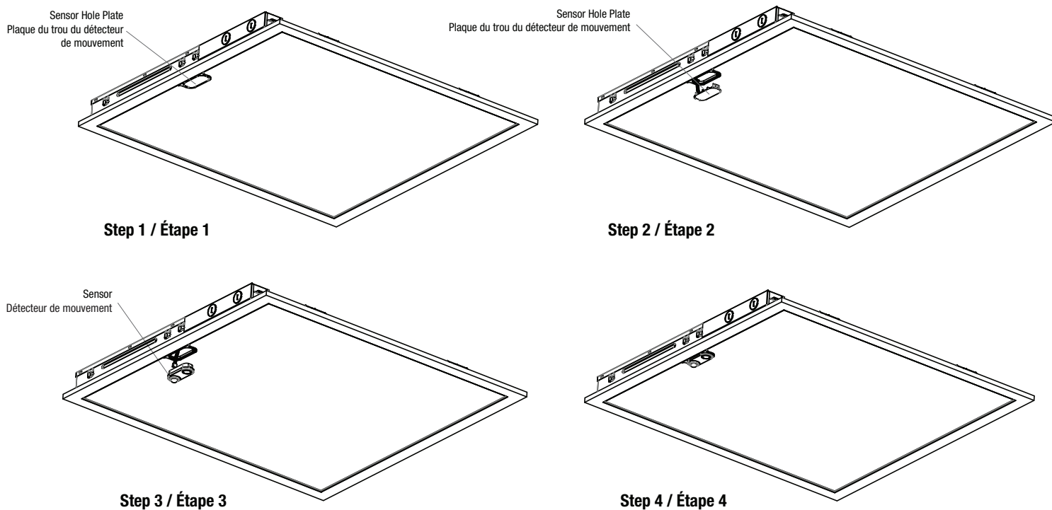
Fig. 4 PIR MOTION SENSOR INSTALLATION (SOLD SEPARATELY) / INSTALLATION DU DÉTECTEUR DE MOUVEMENT IRP (VENDU SÉPARÉMENT)
