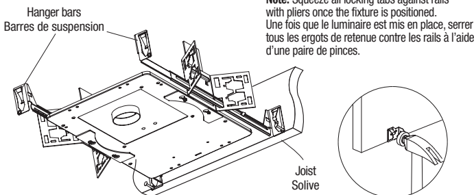
Fig 2 Install hanger bars to the ceiling / Installer les barres de suspension au plafond
