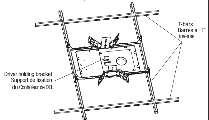
Fig 3 Install hanger bars to T bars ceiling / Installer les barres de suspension au barres en "T" inversé
