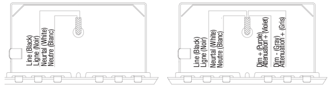
Wiring Diagramme / Schéma de câblage
